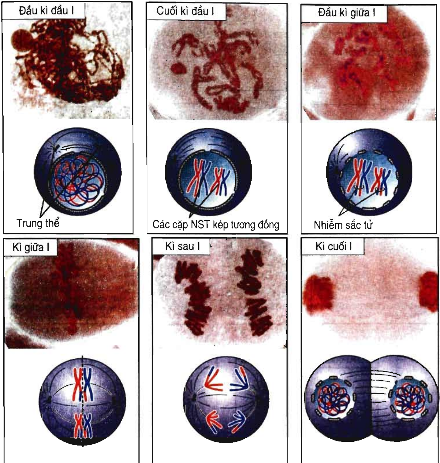
Hình 19.1. Các kì của giảm phân I
