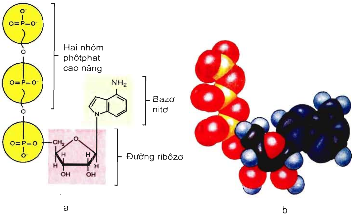
Hình 13.1. Cấu trúc của phân tử ATP
