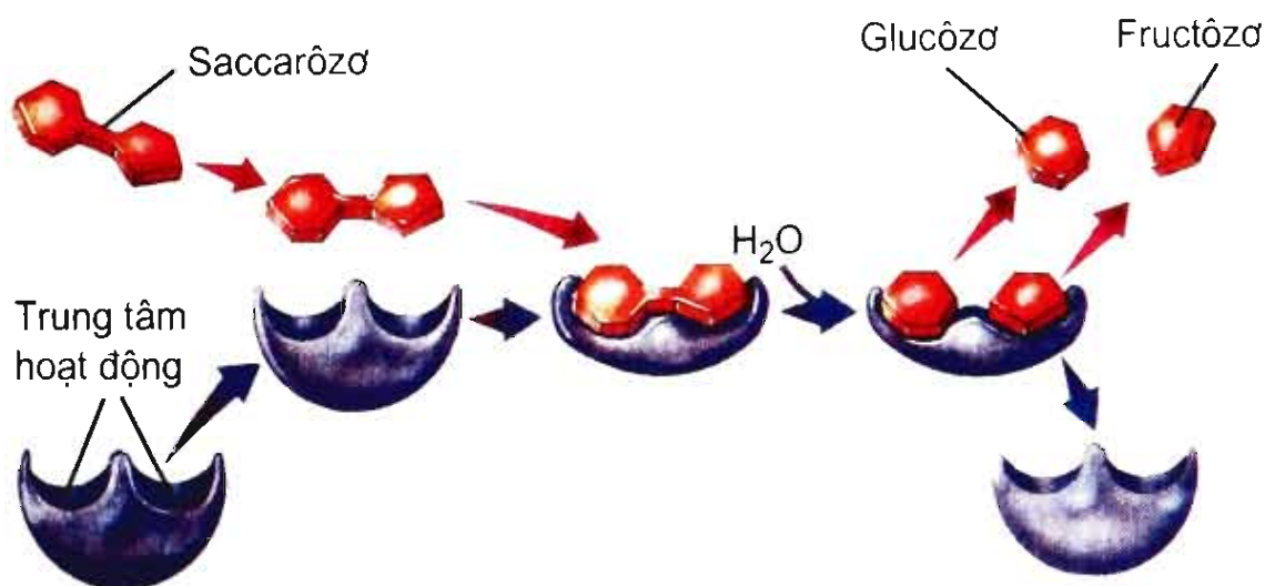
Hình 14.1. Sơ đồ mô tả cơ chế tác động của enzim saccaraza - một loại enzim phân huỷ đường saccarôzơ thành glucôzơ và fructôzơ
