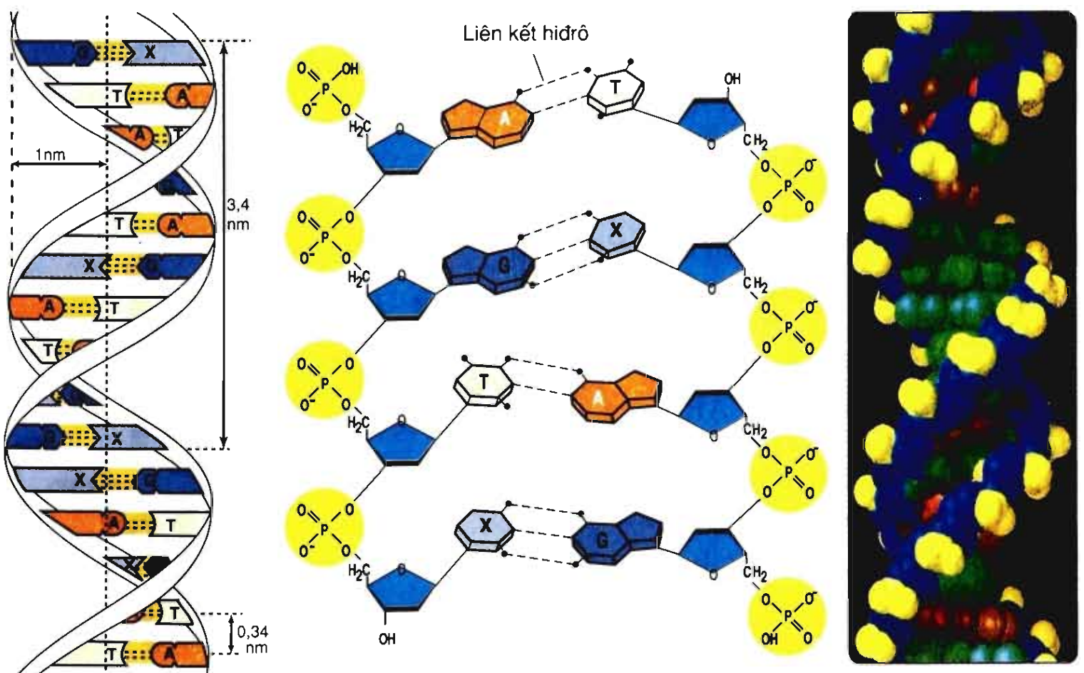
Hình 6.1. Mô hình cấu trúc của phân tử ADN
