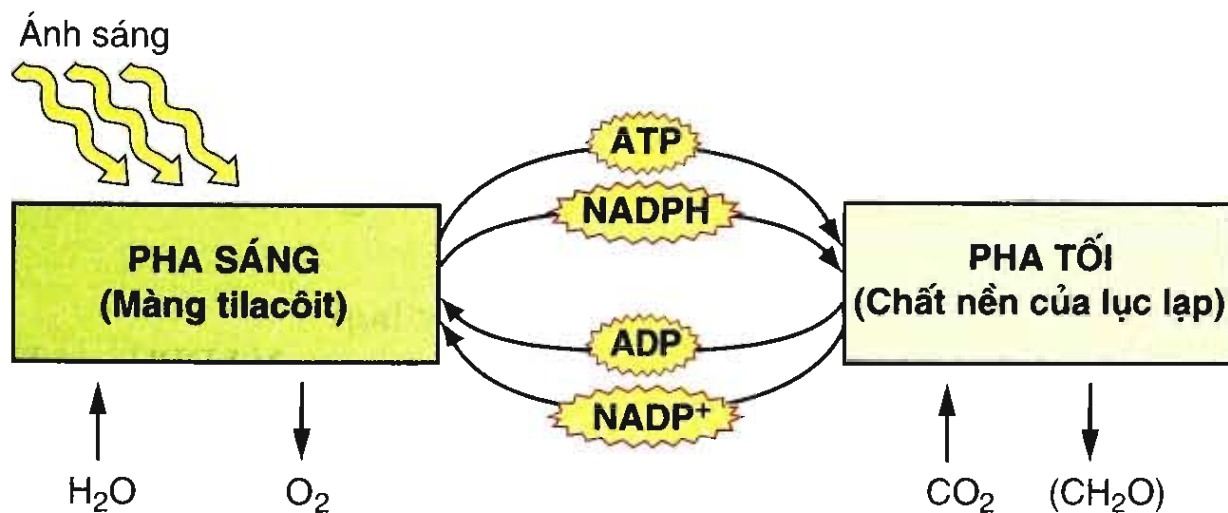
Hình 17.1. Hai pha của quá trình quang hợp
