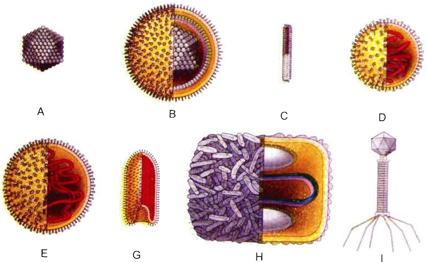
Hình 29.2. Hình thái của một số virut
