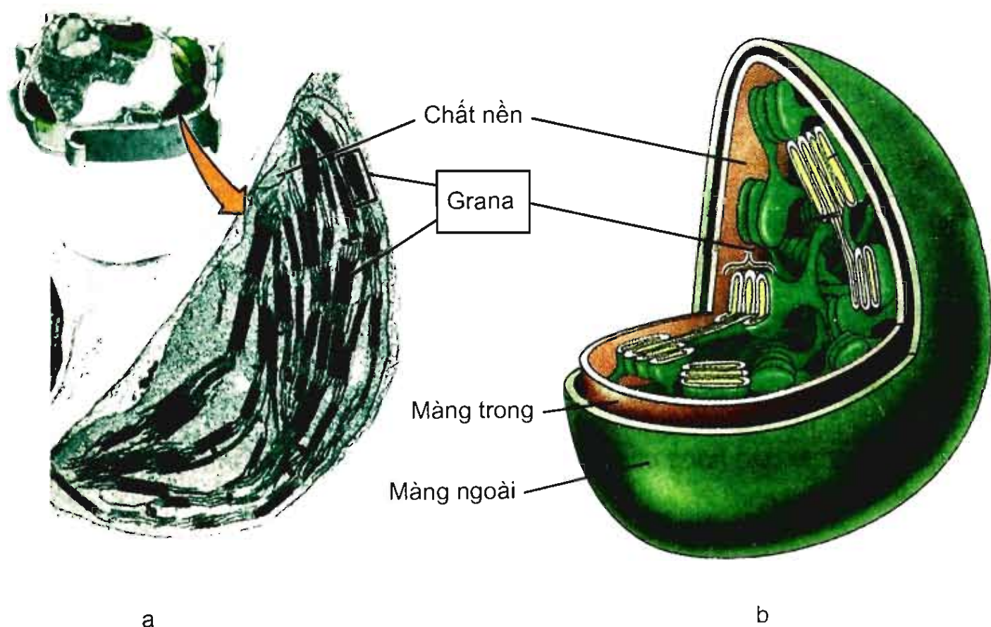
Hình 9.2. Cấu trúc của lục lạp
