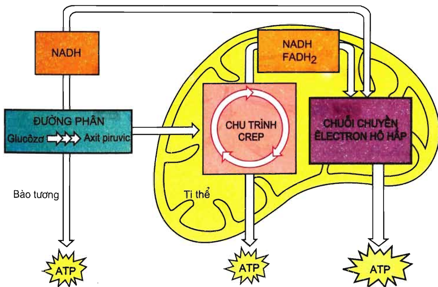
Hình 16.1. Sơ đồ tóm tắt quá trình hô hấp tế bào
