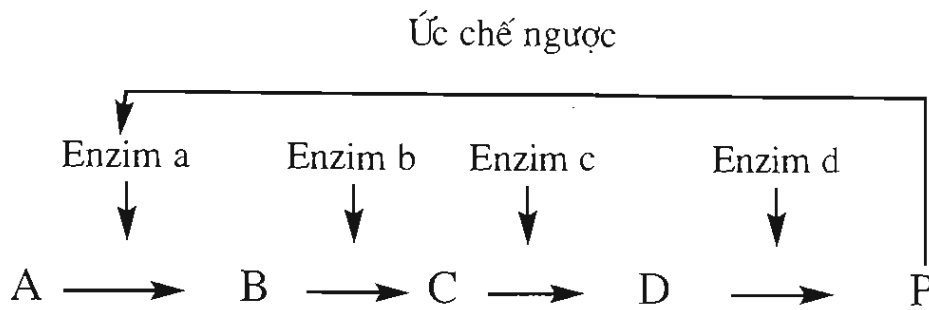
Hình 14.2. Sơ đồ minh họa sự điều hoà quá trình chuyển hoá bằng ức chế ngược.
