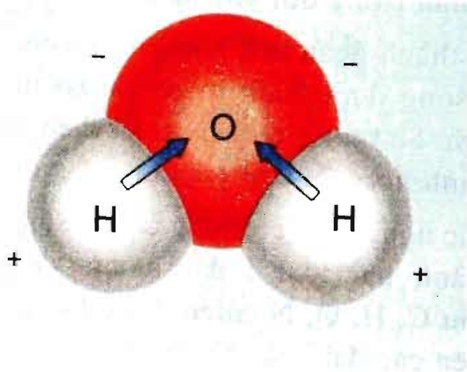
Hình 3.1. Cấu trúc của phân tử nước
