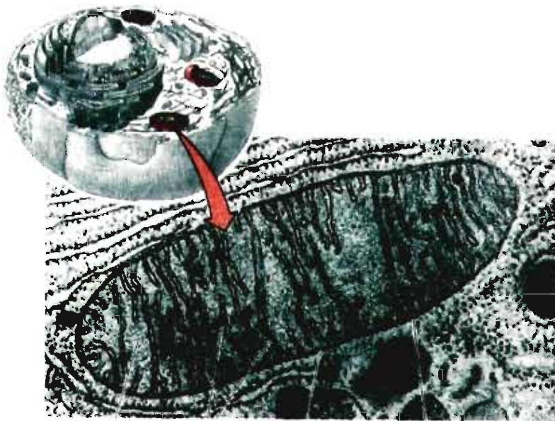
Hình 9.1. Cấu trúc của ti thể
