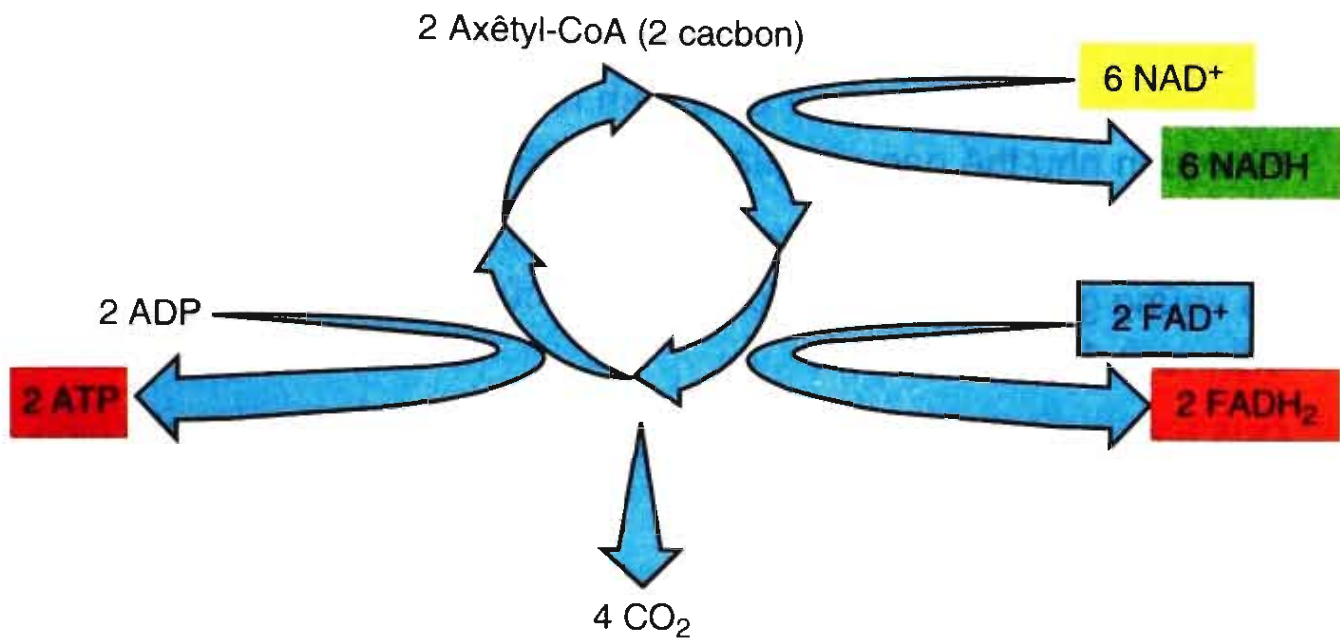
Hình 16.3. Sơ đồ tóm tắt chu trình Crep
