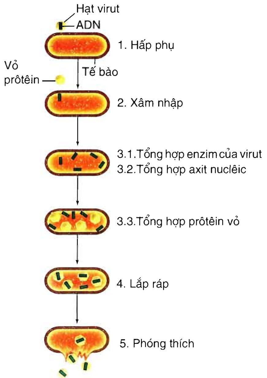
Hình 30. Chu trình nhân lên của phagơ
