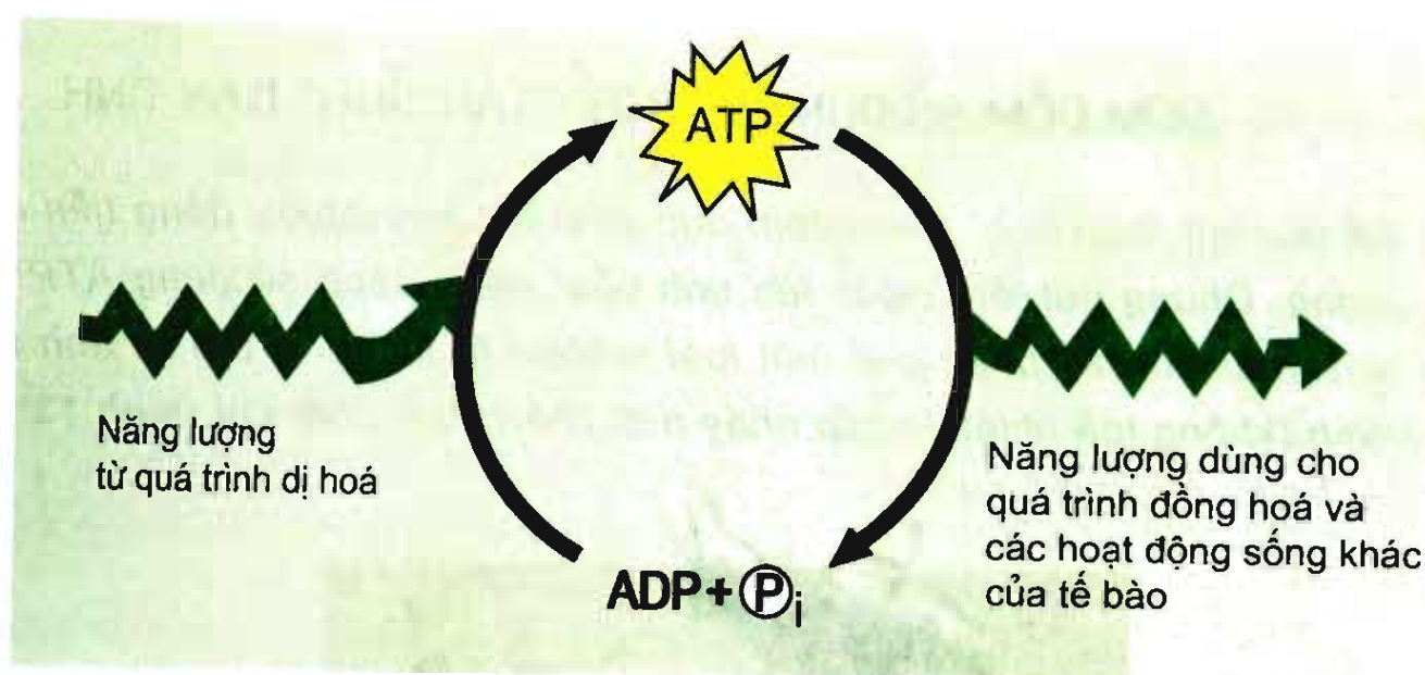
Hình 13.2. Quá trình tổng hợp và phân giải ATP
